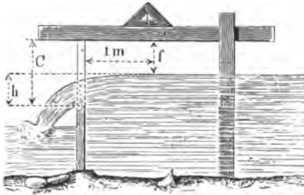
Fig. 6. Überfall.
